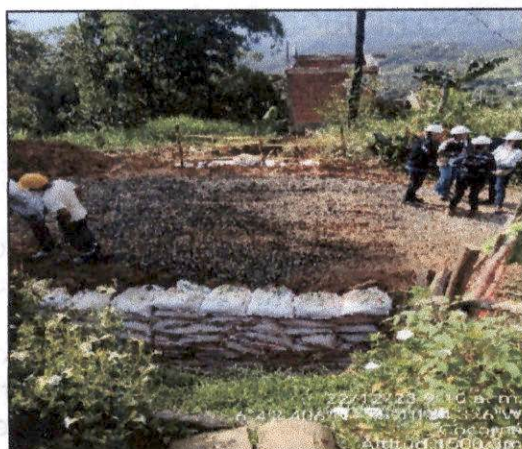
Foto 41 Instalación tubería 900 mm K1+676
