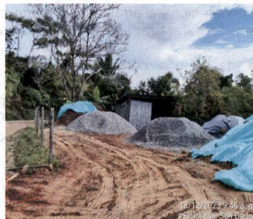
Foto 74. Deposito temporal de materiales pétreos K19+180.
