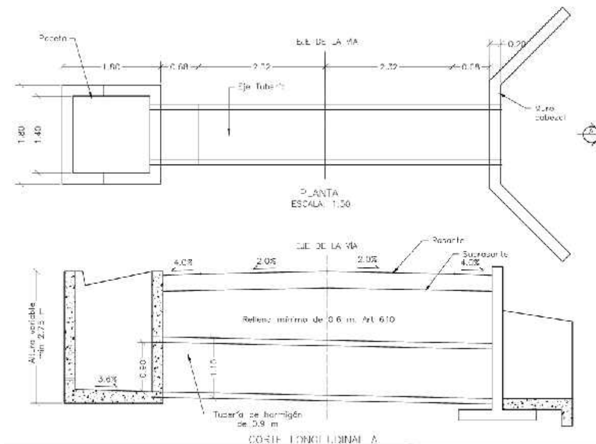
Ilustración 5. Alcantarilla Tipo_Cartilla Obras menores de Drenaje
