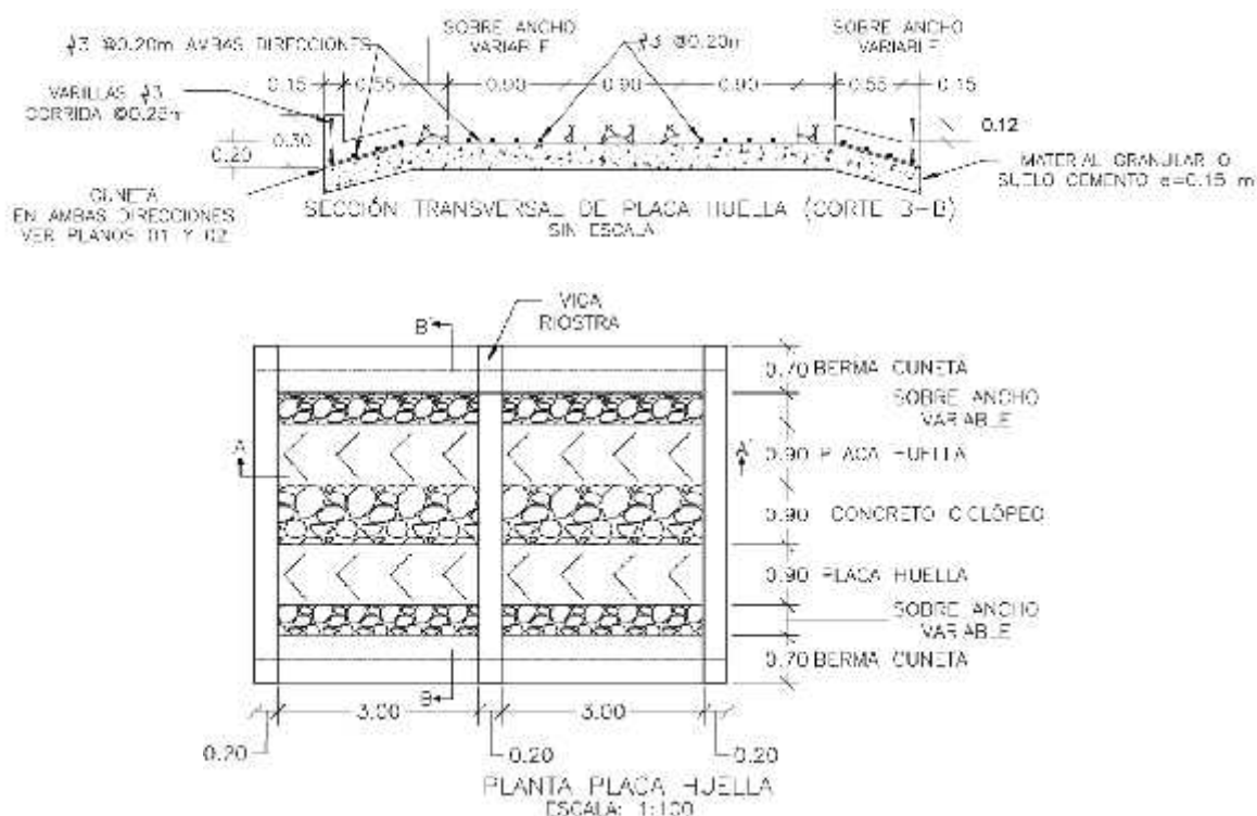
Ilustración 4. Detalle Placa Huella. Fuente: Cartilla Obras menores de Drenaje
