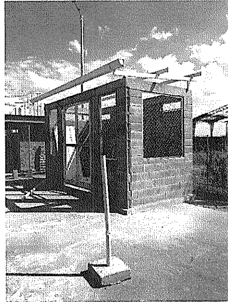
INSTALACIÓN DE PUERTAS Y VENTANAS EN MALLA ESLABONADA.
