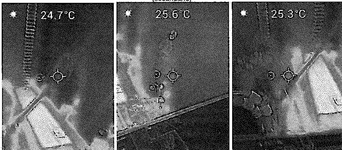
Imagen: Valor máximo medido de temperatura en las conexiones del transformador de salida del UPS
