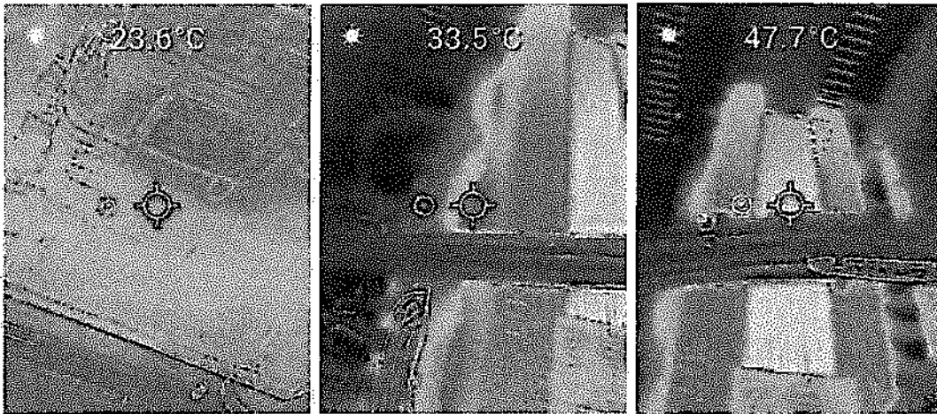
Imagen: Valores de temperatura en los transformadores de entrada y salida del UPS (Máximo-Medio-Mínimo)
