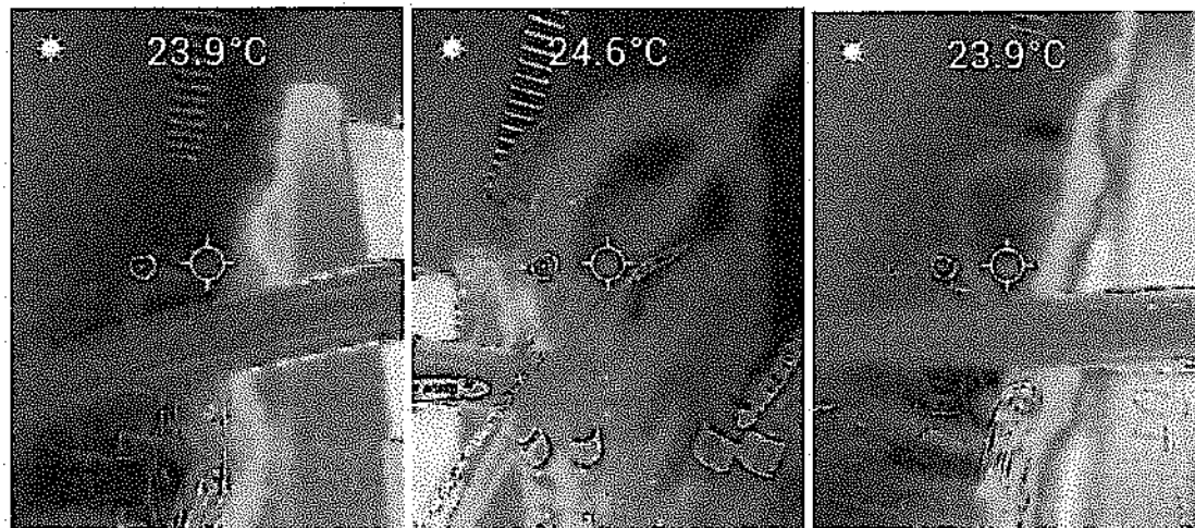
Imagen: Valor máximo medido de temperatura en las conexiones del transformador de entrada del UPS (secundario)
