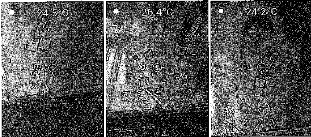
Imagen: Valor máximo medido de temperatura en las conexiones del transformador de entrada del UPS (primario)
