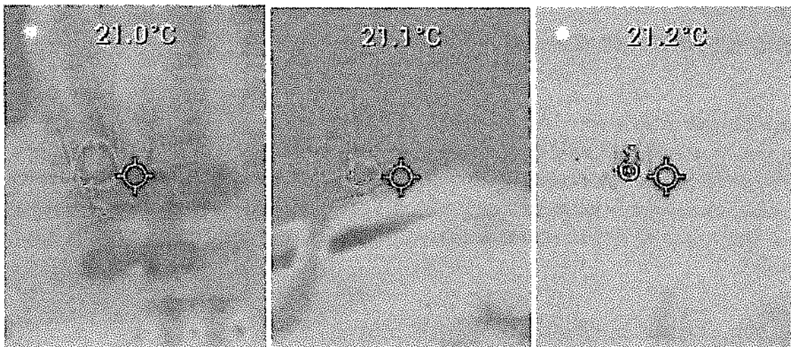
Imagen: Valor máximo medido de temperatura en protección de entrada de UPS 150KVA.
