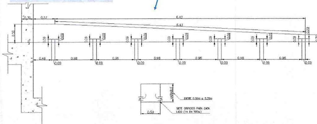
TRES UNIDADES POR CEDIMENTADOR MULTIPLE DISTRIBUIDOR DE AGUA FLOCULADA DETALLE 07 - PTAP ESCALA: 1:25
