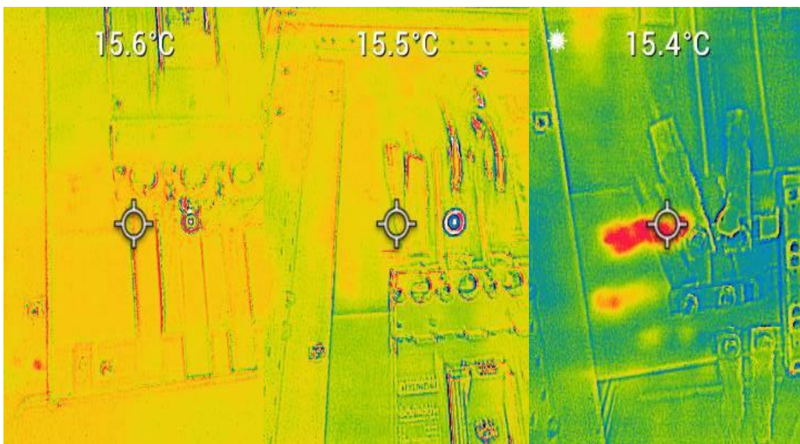
Imagen: Valor máximo medido de temperatura en protección de UPS 150KVA
