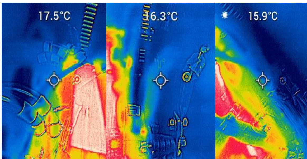
Imagen: Valor máximo medido de temperatura en las conexiones del transformador de entrada del UPS
