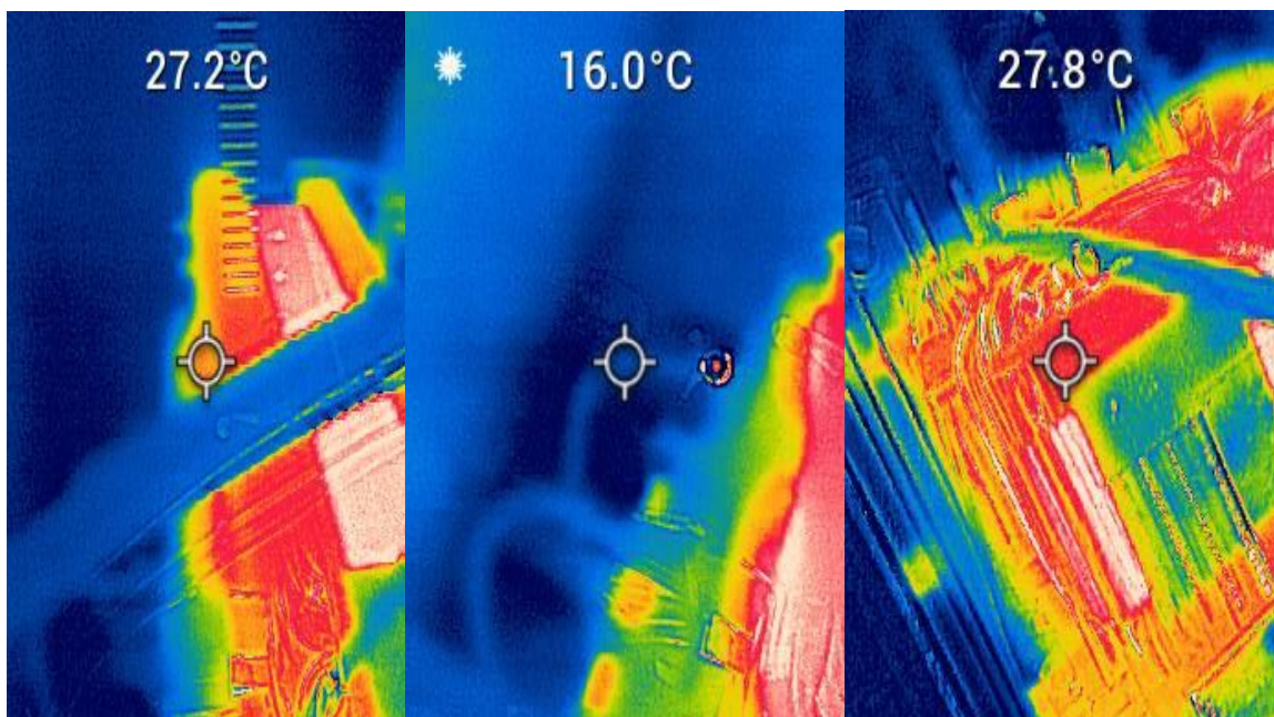
Imagen: Valores de temperatura en los transformadores de entrada y salida del UPS
