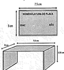
Ilustración 1 - Placa utilizada para identificación de Vértices Geodésicos
