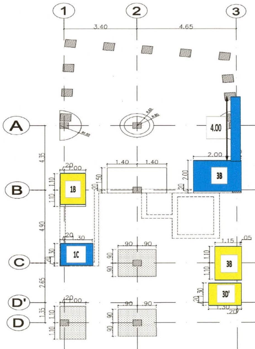
PLANTA DE CIMENTACIÓN, UBICACIÓN MURO DE SUBMURACIÓN
