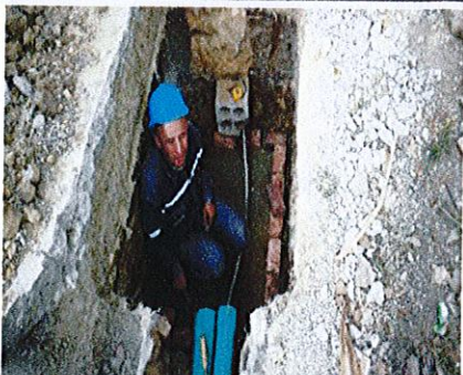
FOTO No. 11 CIV 16002846 - Construcción de caja de paso para red de ETB costado oriental carrera 32C.
