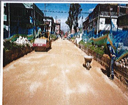
FOTO No. 9 CIV 16002879 y CIV 16002905 - Compactación de primera capa de subbase 0,15cm.
