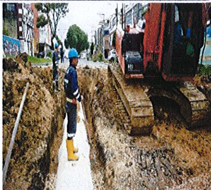
FOTO No. 11 CIV 16002905 - Excavación mecánica para estructura de pavimento. Red 30" aguas lluvias.
