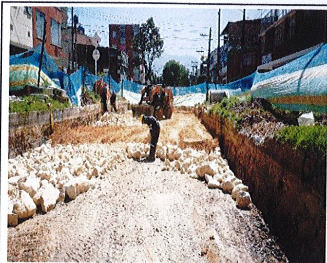
CIV 16002905 - Extendido de capa granular para sello de rajón.
