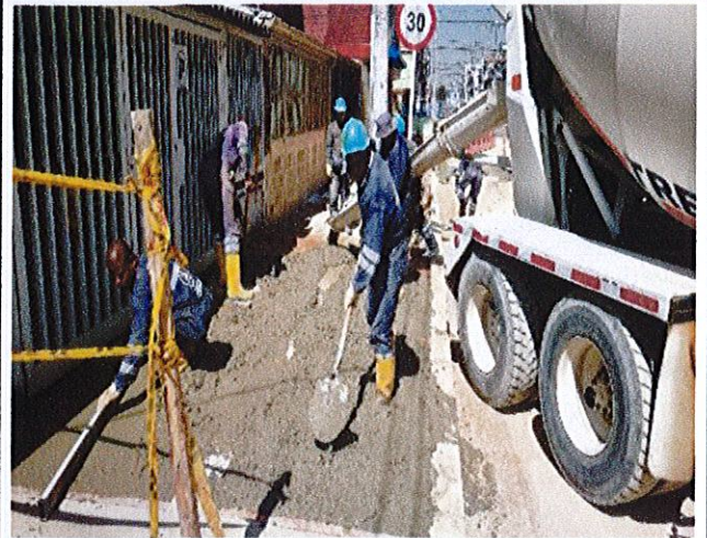
CIV16002769 - Fundida de placa de pavimento rígido MR-45, colocación de aceros de refuerzo y acero de transferencia.
