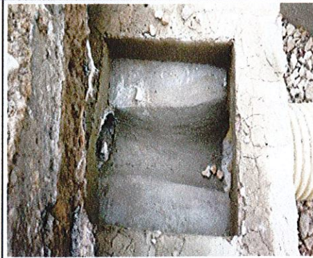
FOTO No. 12 CIV 16002879 - Construcción de cajas de paso redes lluvias, sumideros existentes carrera 32A.
