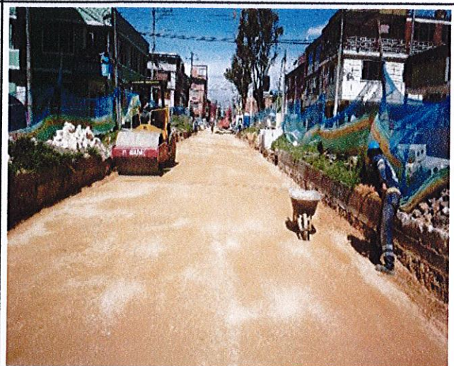
CIV 16002879 - Compactación de primera capa de subbase 0,15cm.
