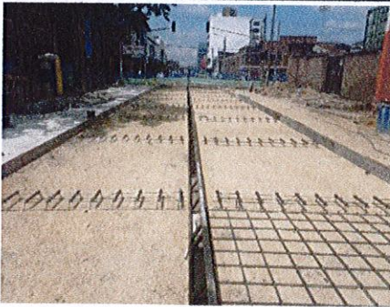
FOTO No. 1 CIV 16001745 - Instalación canastillas con barras de transferencia de carga y acero de refuerzo para losas.
