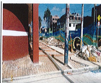
FOTO No. 12 CIV 16002905 - Alistamiento de zona de andén, limpieza e instalación de malla electrosoldada.
