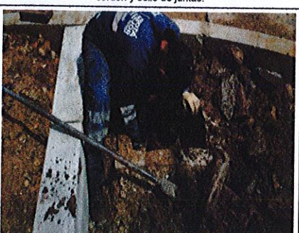
FOTO No. 6 CIV 16002879 - Limpieza de caja válvula esquina sur oriental cruce carrera 32A.
