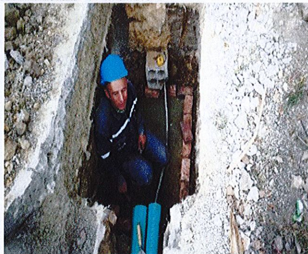
CIV 16002846 - Construcción de caja de paso para red de ETB costado oriental carrera 32C.
