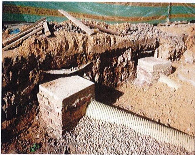
CIV 16002879 - Construcción de cajas de paso red de aguas lluvias.
