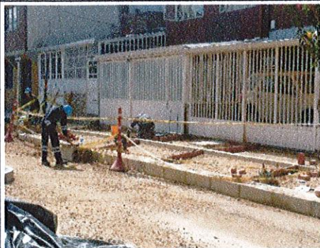
FOTO No. 7 CIV 16002769 - Construcción de cenefas para dilatación de placas de concreto.
