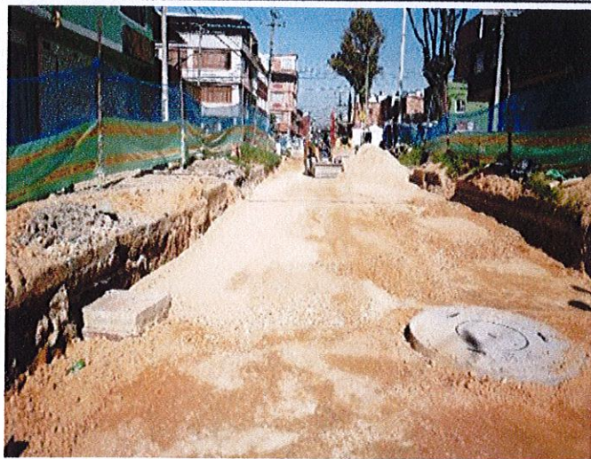
CIV 16002879 - Extendido de capa granular primera capa.
