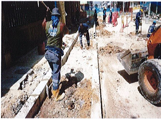
CIV16002769 - Excavación manual para conformación de andenes.
