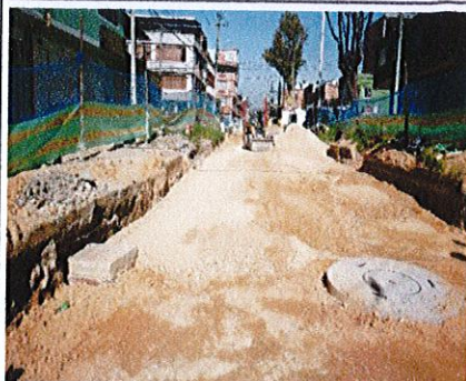
FOTO No. 8 CIV 16002879 - Extendido de capa granular primera capa.
