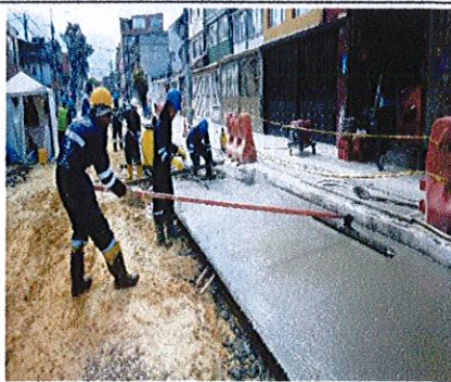
FOTO No. 5 CIV 16002769 - Aplicación de retardante de evaporación y rallado de superficie.
