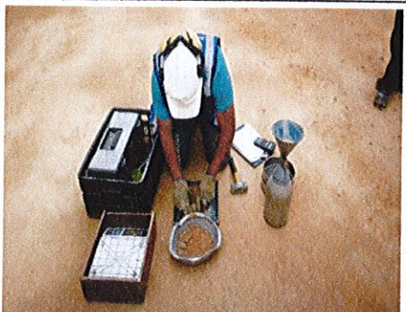
FOTO No. 10 CIV 16002879 y CIV 16002905 - Toma de densidades al material granular.
