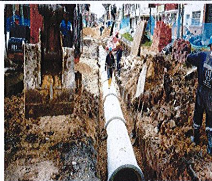
FOTO No. 5 CIV 16002769 - Instalación tubería concreto reforzado 30" red aguas lluvias.
