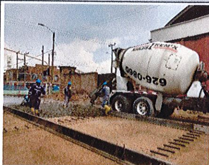
FOTO No. 2 CIV 16001745 - Construcción de losas de concreto Costado Norte Interior
