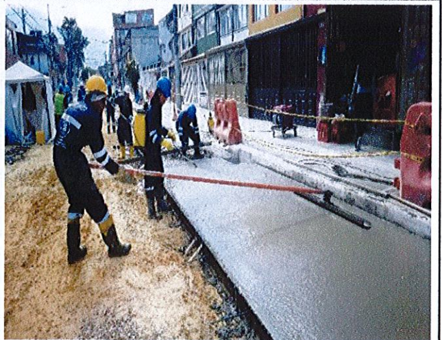
CIV 16002769 - Aplicación de retardante de evaporación y rallado de superficie.
