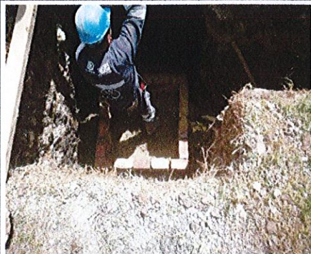
FOTO No. 10 CIV 16002905 - Construcción caja domiciliaria red sanitaria, costado norte.
