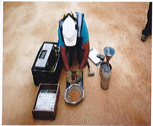
CIV 16002879 - Toma de densidades al material granular.
