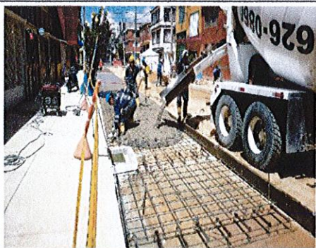
FOTO No. 4 CIV 16002769 - Fundida de placa de pavimento rígido MR-45, colocación de aceros de refuerzo y acero de transferencia.
