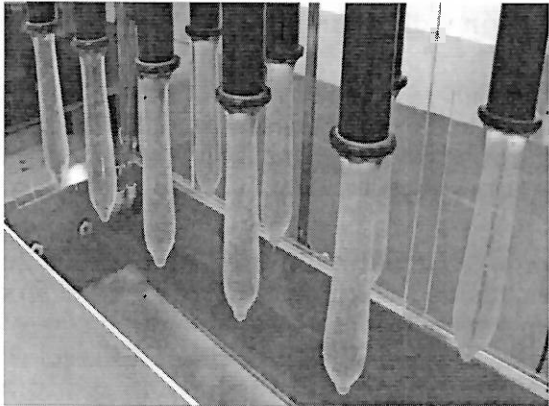
Equipo para prueba de detección de orificios en preservativos masculinos de látex.
