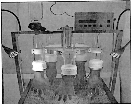
Equipo para prueba de impermeabilidad en guantes
