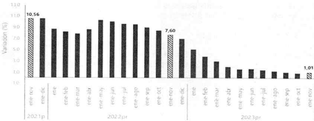
Gráfico 7. Tasa de crecimiento año corrido del índice del Indicador de Seguimiento a la Economía (ISE) Serie original 2021p - 2023pr (enero-noviembre)
