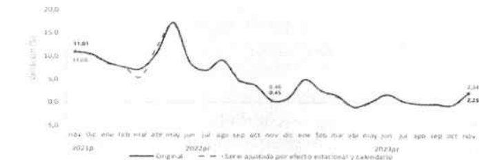
Gráfico 1. Tasa de crecimiento anual del índice del Indicador de Seguimiento a la Economía (ISE) Serie original y serie ajustada por efecto estacional y calendario 2021p - 2023pr (noviembre)
