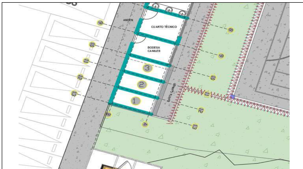
Reubicación de canales
