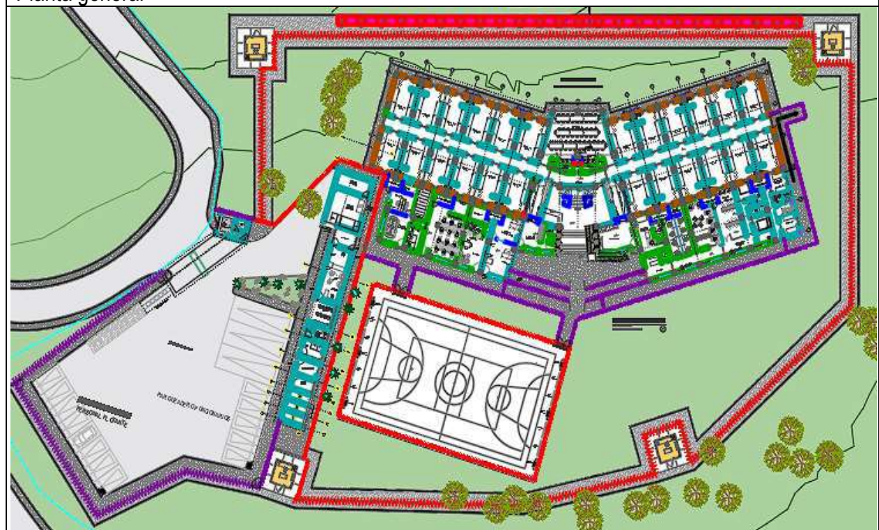
Planta general primer nivel
