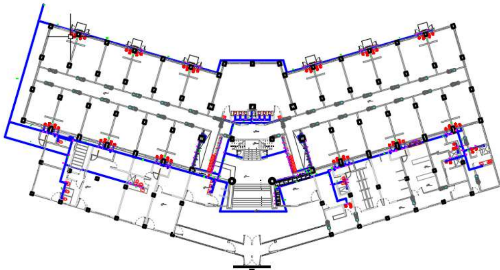
Red de abastos primer piso
