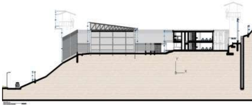
Ilustración 4. Corte SECCION A-A
