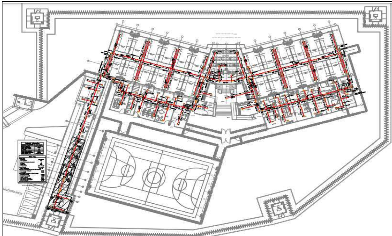
Diseño de red contra incendio.
