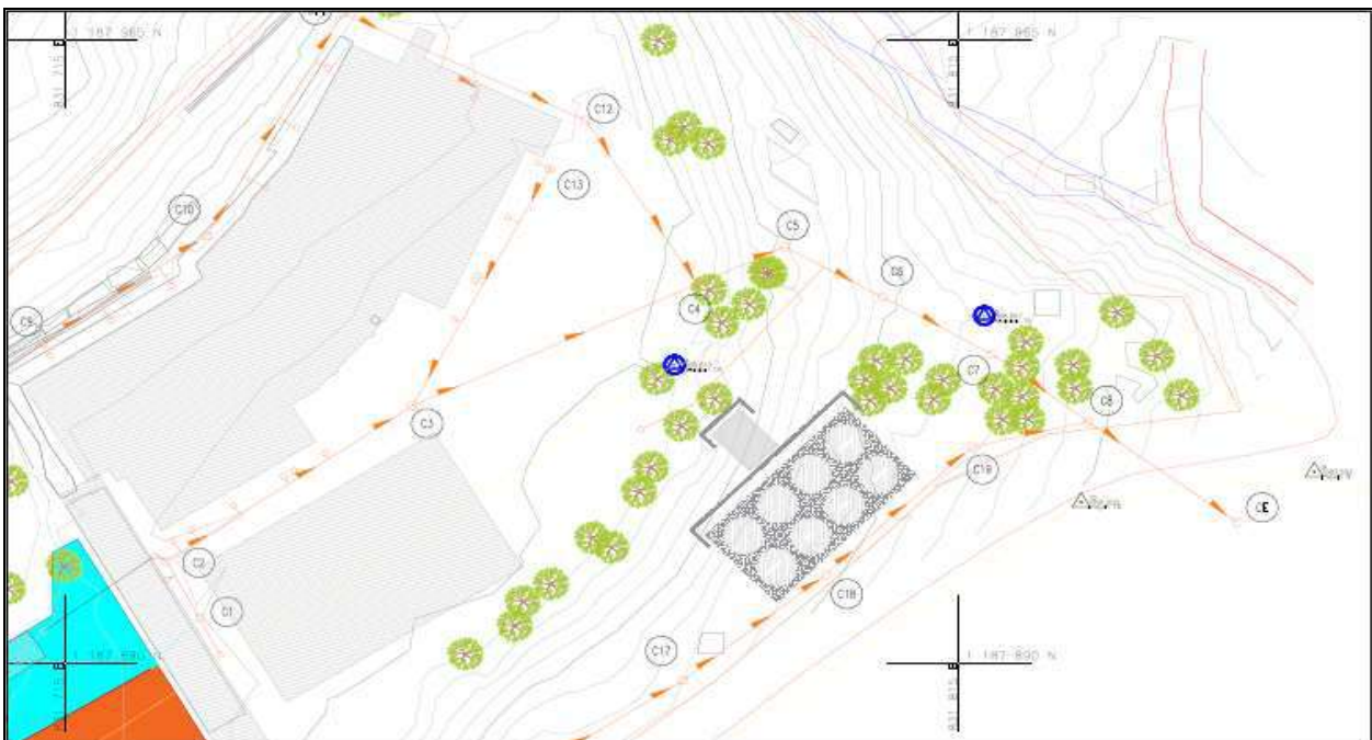
Diseño red alcantarillado
