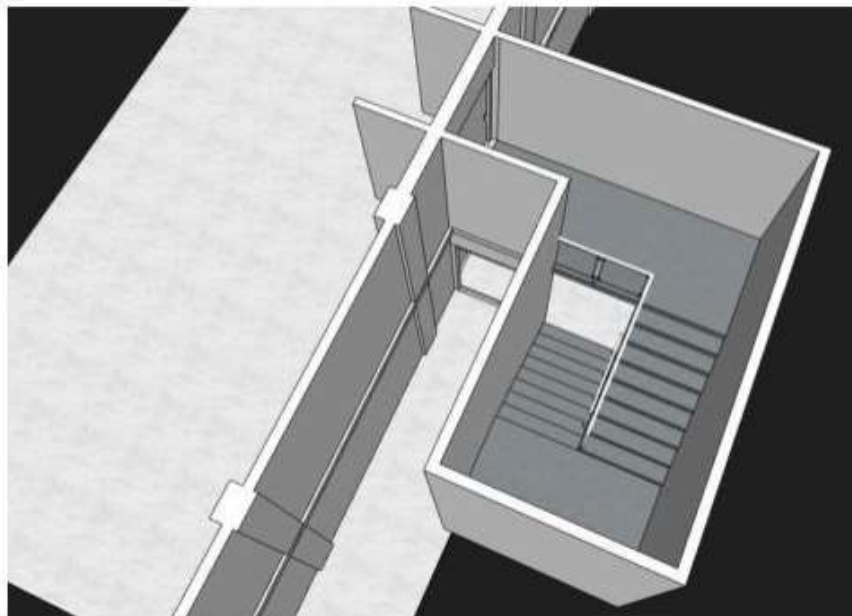
Ilustración 12. Vista en 3D de escaleras de emergencia segundo nivel Centro de Reclusión AURES
