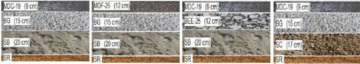
Alternativas en la estructura del pavimento flexible planteadas.
