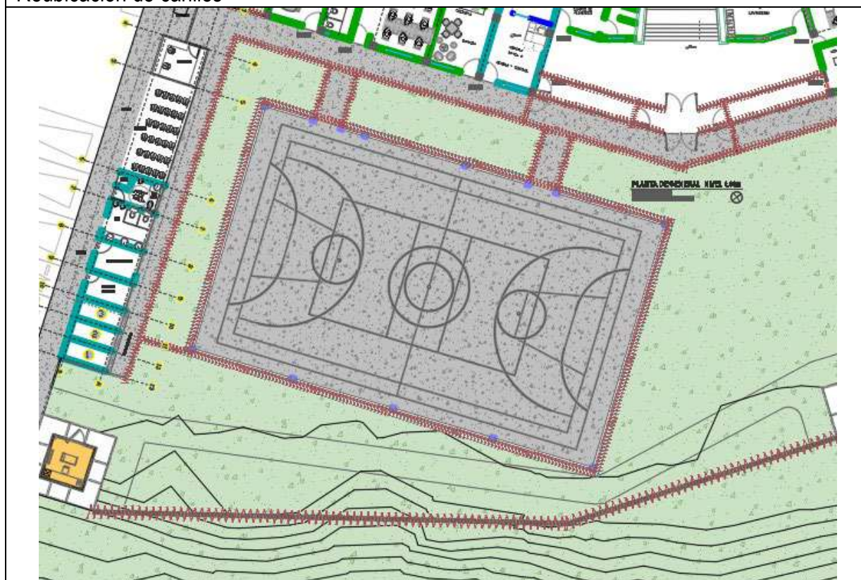
Diseño de cerramiento
