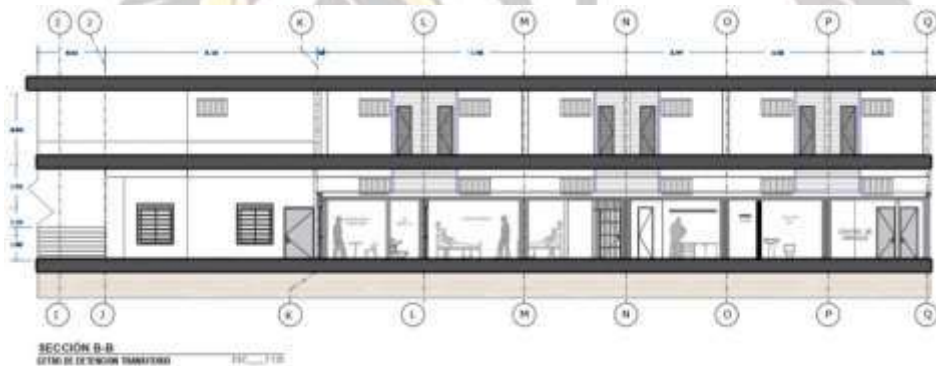
Ilustración 1. Corte SECCION B-B
