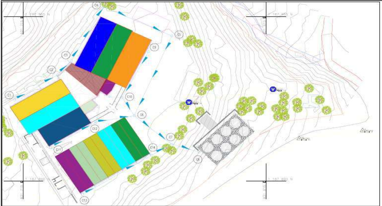
Diseño tramo red de circulación
