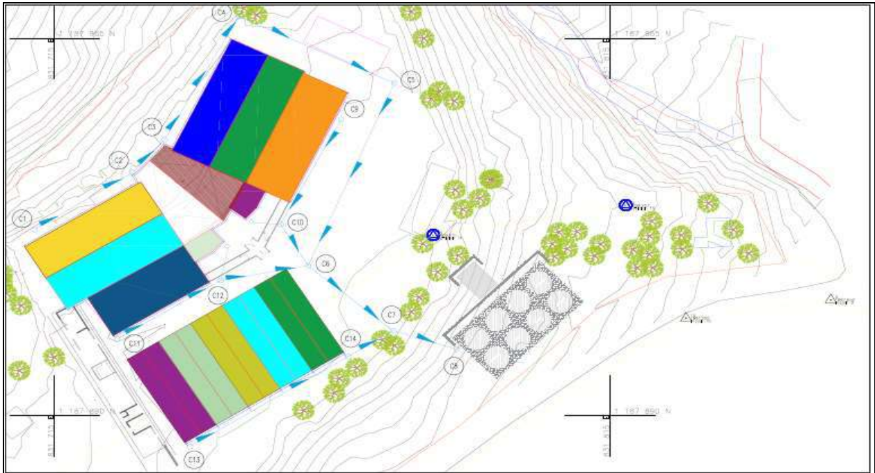
Red de recolección de aguas lluvias
