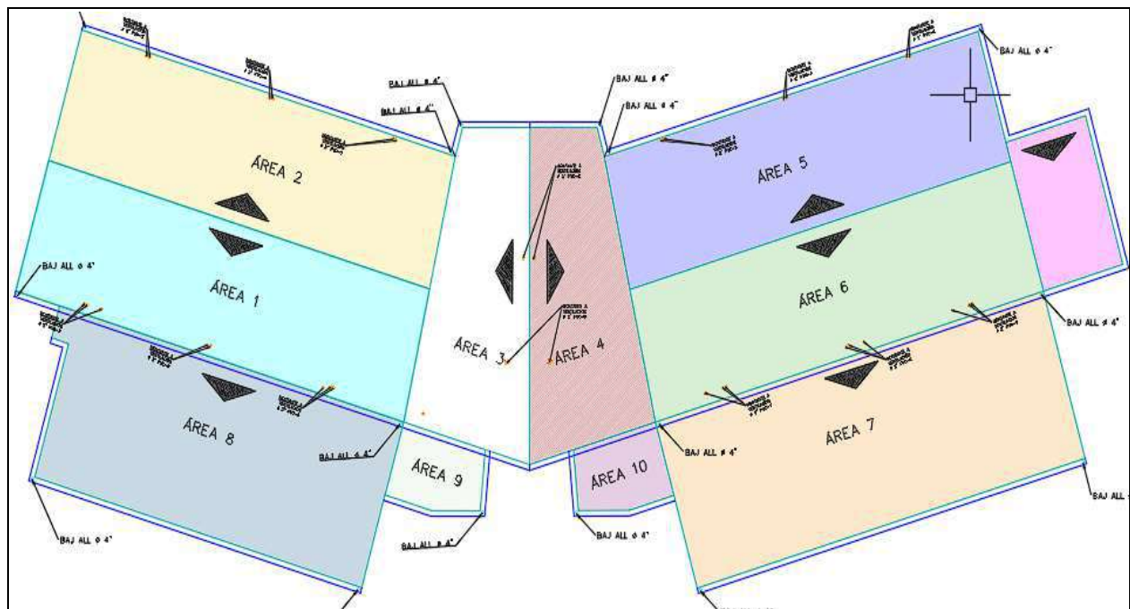
Planta cubiertas, canoas y bajantes
