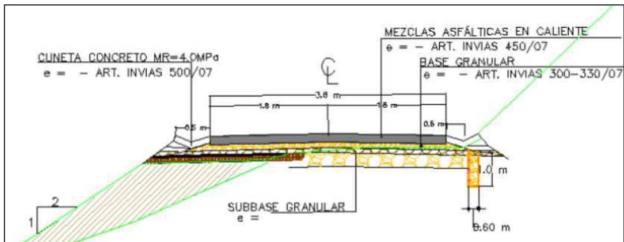
Diseño sección transversal.
