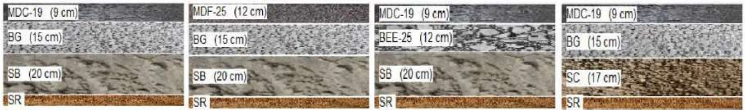
Alternativas en la estructura del pavimento flexible planteadas.
