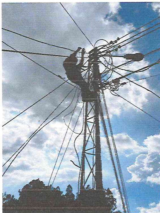
Conexión de acometida eléctrica a poste principal
