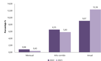
Gráfico 1. IPC Variaciones Total, Nacional Mayo 2022 - 2023
