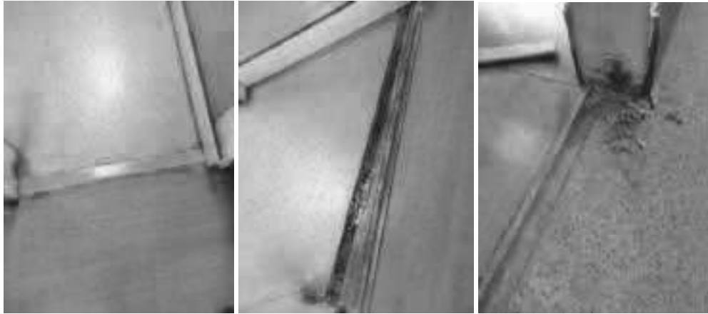
(Otros – Piso - Pirlan) Cambio de pirlan (reductor piso laminado), piso N° 3 – Occidente – Antigua sala 3-4.
