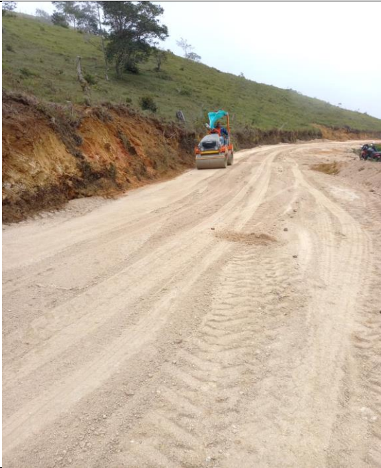
Instalación de subbase granular
