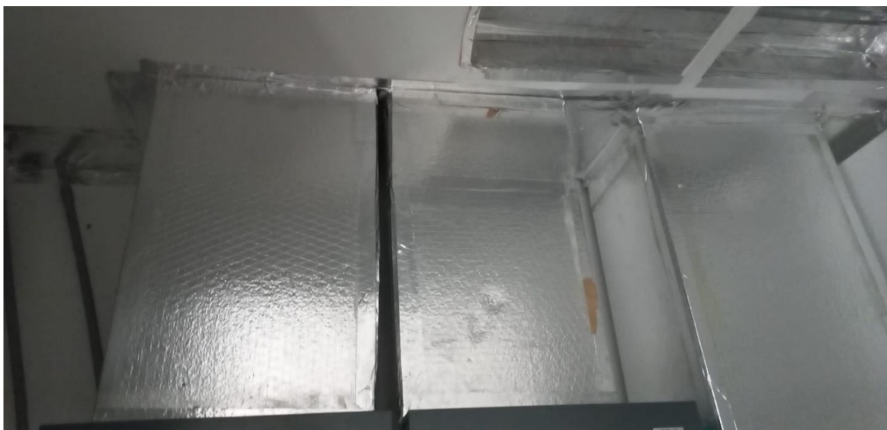
EMPALME DE DUCTO EN LAS (3) MANEJADORAS
