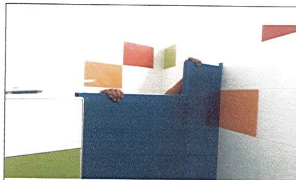
INSTALACIÓN DE PUERTAS METALICAS PARA SANITARIOS
