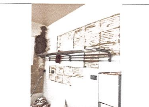
DESMONTE DE ENCHAPES FISURADOS DE MURO
