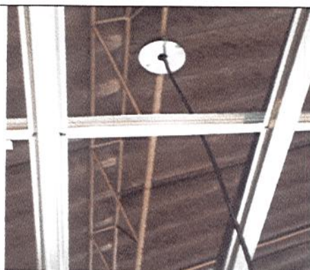
INSTALACION DE ESTRUCTURA PARA CIELO RASO EN SUPERBOARD EN SALONES Y RED ELECTRICA
