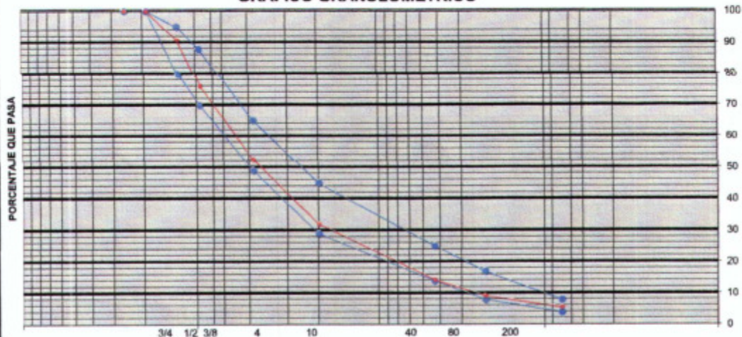
GRÁFICO GRANULOMÉTRICO
