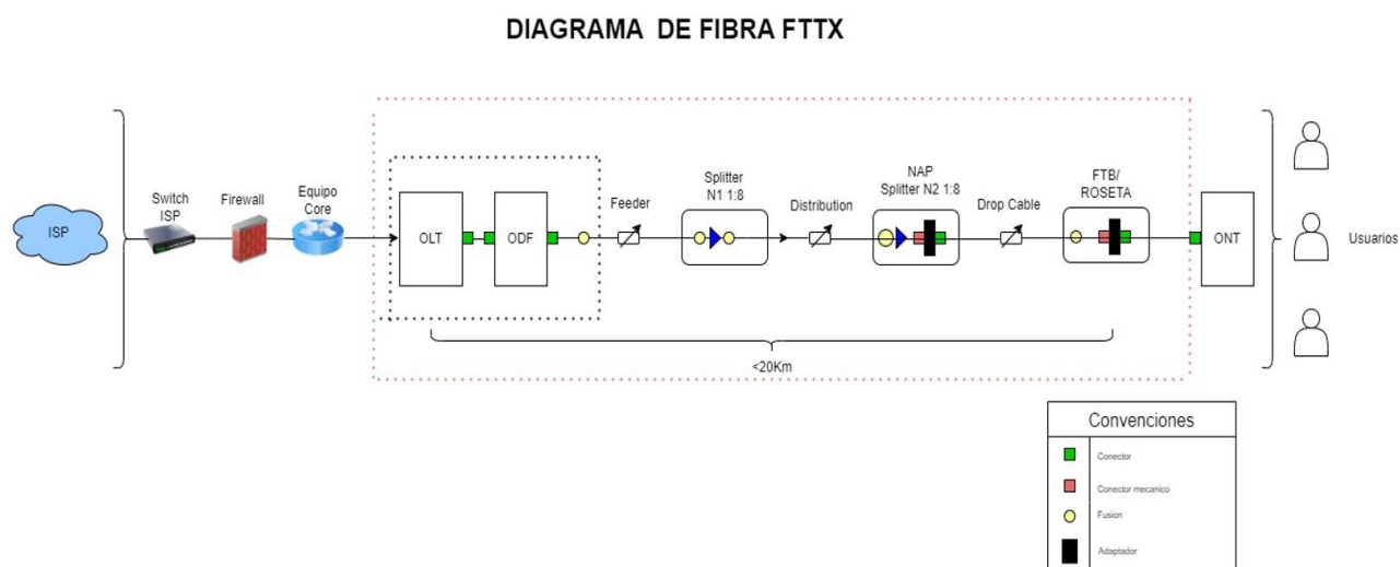
Ilustración 3 Diagrama de Fibra FTTX
