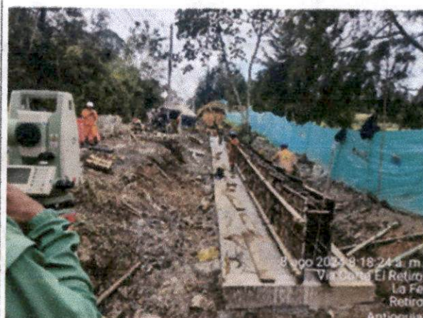
Foto N°12. Chequeo topográfico de alineamiento de vástago, marcación de niveles de terminado y levantamiento de la excavación realizada muro N°5
