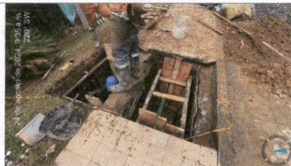
Foto N°37. Instalación de tubería sanitaria K2+195 – K2+230
