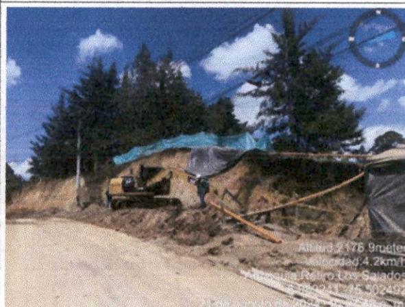
Foto N°28. Excavaciones y perforación de micropilotes para construcción de muro K1+900 muro de contención N°5
