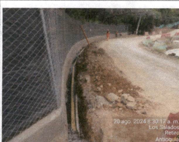
Foto N°37. Instalación de tubería sanitaria K2+195 – K2+230
