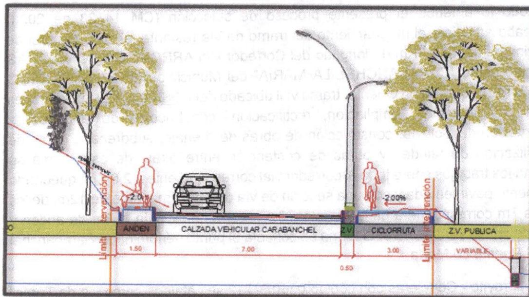
Ilustración 1. sección vial del proyecto
