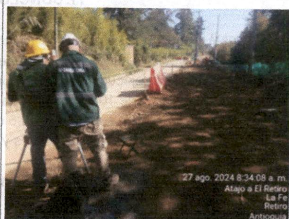
Foto N°54. Chequeo y marcación topográfica de sumidero sobre ciclorruta K2+280 - K2+360
