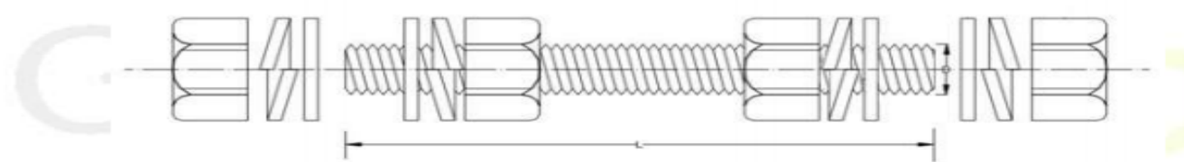
Figura 1 Geometría y dimensiones del espárrago
