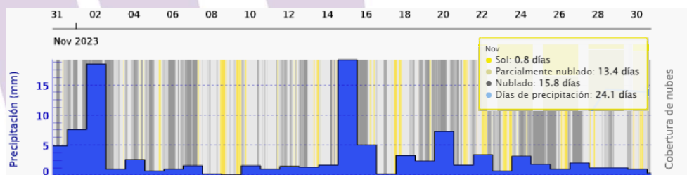
Imagen 10. Precipitación en El Bordo Mes de Noviembre. Fuente www.meteoblue.com.es
