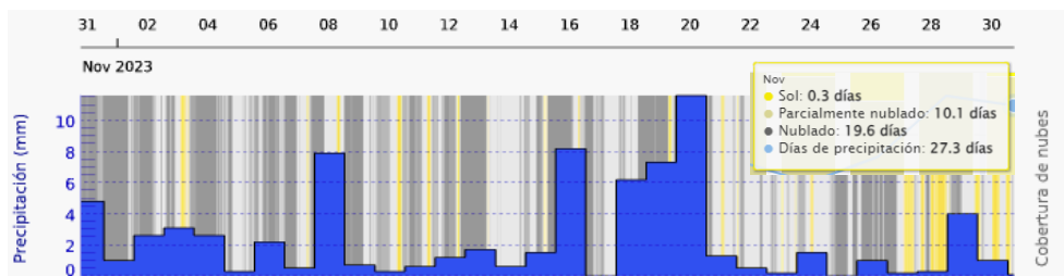
Imagen 4. Precipitación en Pereira Mes de Noviembre. Fuente www.meteoblue.com.es
