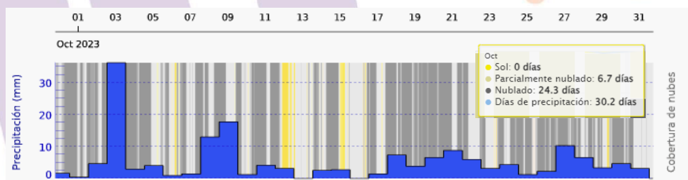
Imagen 1. Precipitación en Frontino Mes de Octubre. Fuente www.meteoblue.com.es
