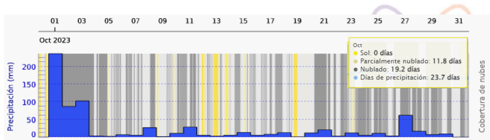
Imagen 11. Precipitación en Istmina Mes de Octubre. Fuente www.meteoblue.com.es
