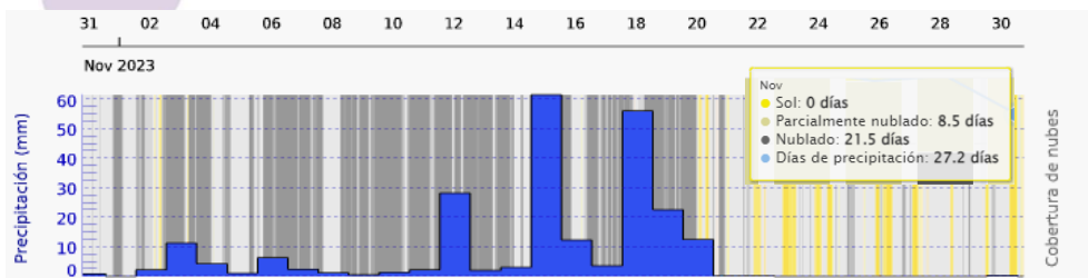
Imagen 2. Precipitación en Frontino Mes de Noviembre. Fuente www.meteoblue.com.es
