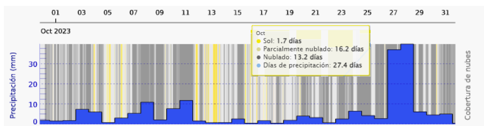
Imagen 7. Precipitación en Sevilla Mes de Octubre. Fuente www.meteoblue.com.es
