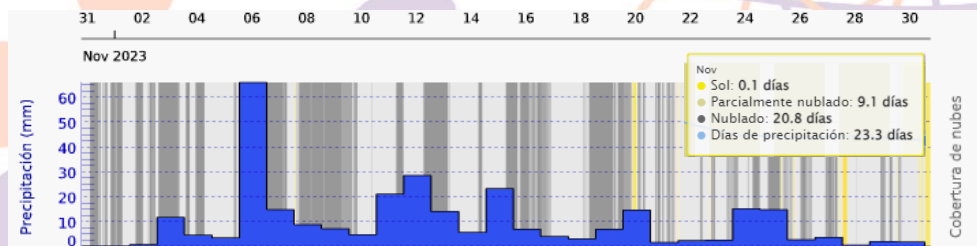
Imagen 12. Precipitación en Istmina Mes de Noviembre. Fuente www.meteoblue.com.es
