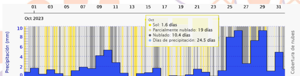
Imagen 9. Precipitación en El Bordo Mes de Octubre. Fuente www.meteoblue.com.es
