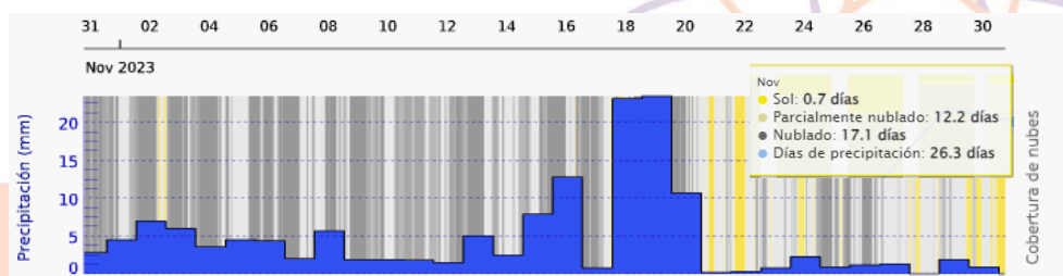
Imagen 8. Precipitación en Sevilla Mes de Noviembre. Fuente www.meteoblue.com.es
