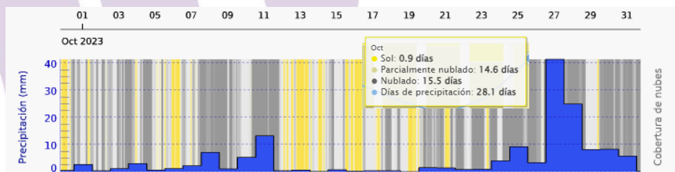
Imagen 3. Precipitación en Pereira Mes de Octubre. Fuente www.meteoblue.com/es
