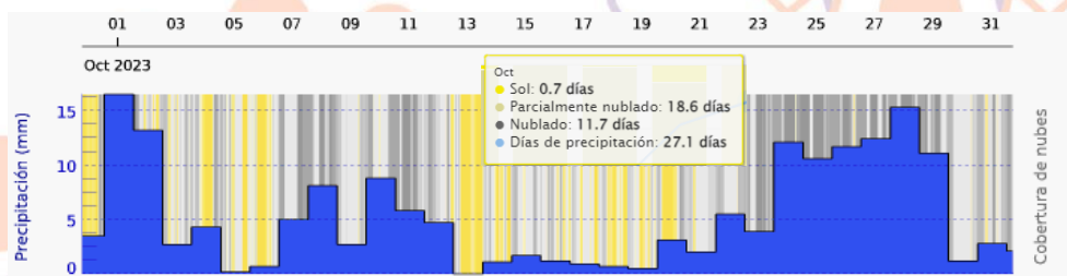
Imagen 5. Precipitación en Cali Mes de Octubre. Fuente www.meteoblue.com.es
