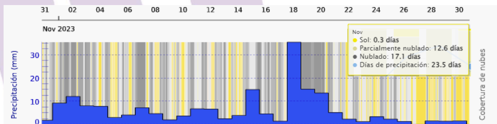
Imagen 6. Precipitación en Cali Mes de Noviembre. Fuente www.meteoblue.com.es
