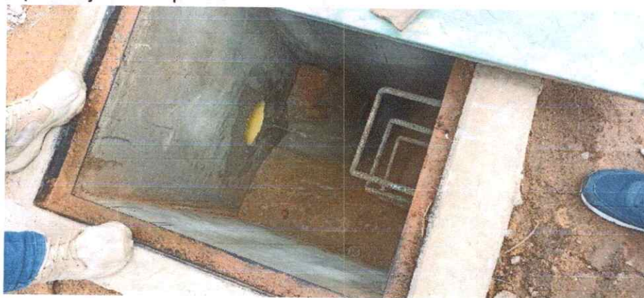
Peldaños para cajas de inspección
