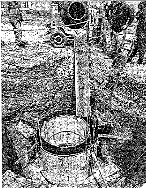
Fundida de manhol.
