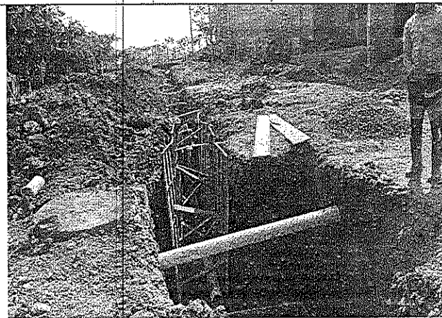
Entibado en instalación de alcantarillado.
