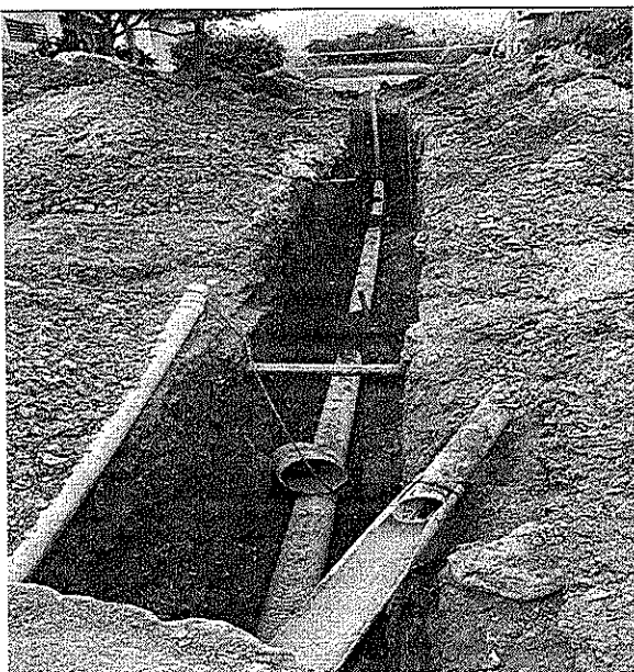
Instalacion de tuberia de alcantarillado.
