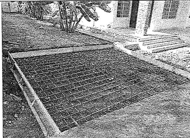
Acero de refuerzo de bocacalles
