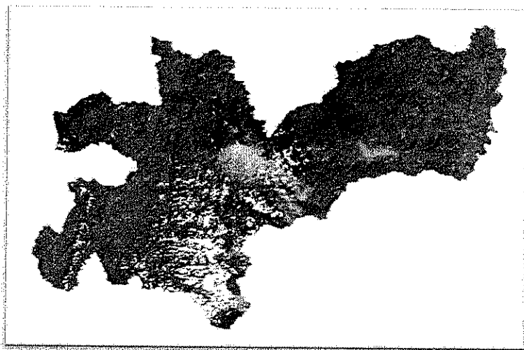
Imagen 2: Imagen LandSat 8 del año 2015 donde se nota la cobertura vegetal para ese año de color verde oscuro.
