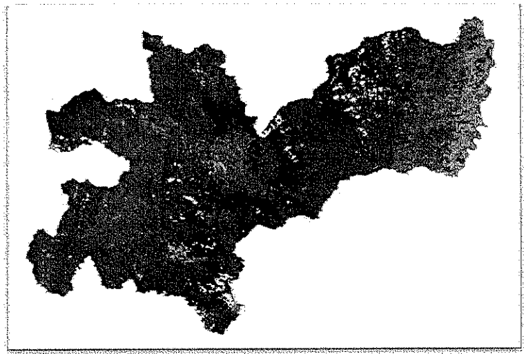
Imagen 3: Imagen LandSat 8 del año 2019 donde se aprecia la cobertura vegetal de color verde oscuro.
