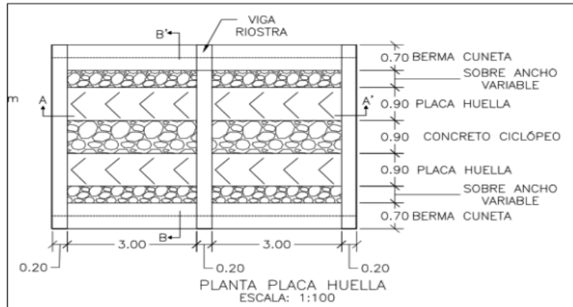
Imagen 5. Planta Placa Huella
