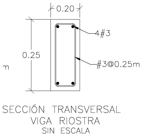
Figura 4 Esquema Sección viga riostra
