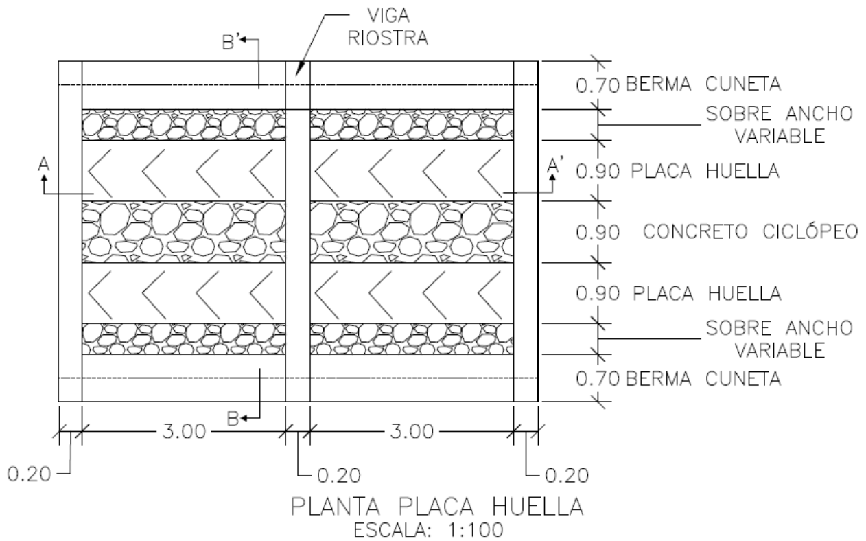
Figura 2 Esquema Vista en planta
