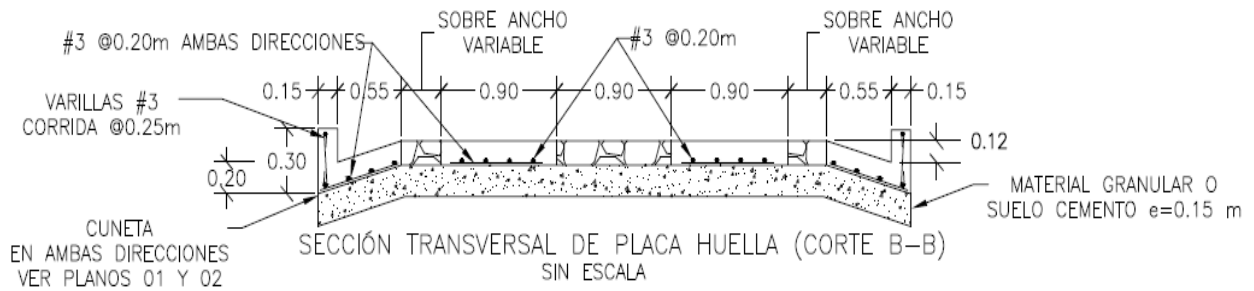
Figura 1 Esquema placa huella sección transversal
