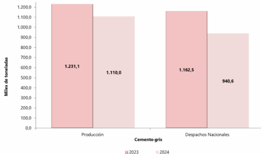
Gráfico 1. Producción y despachos de cemento gris (miles de toneladas) Total nacional Marzo (2023 – 2024 Pr )
