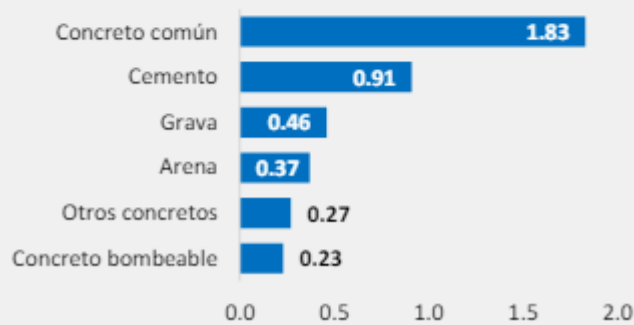
Gráfica 1.6: ICOCED – Materiales según principales insumos. Ponderación sobre el total del ICOCED en porcentaje - octubre 2023
