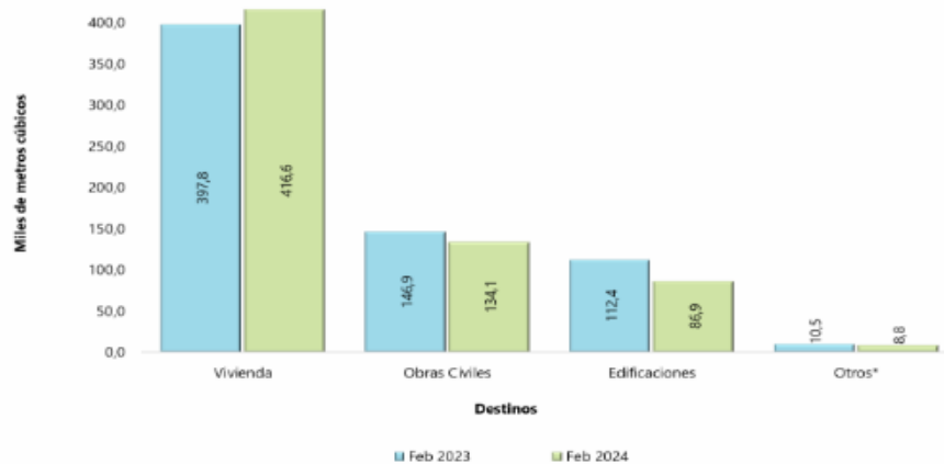
Gráfico 1. Producción de concreto premezclado según destinos (miles de metros cúbicos) Total nacional Febrero (2023-2024 P )
