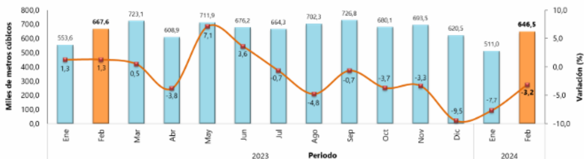
Gráfico 2. Producción de concreto premezclado (miles de metros cúbicos y variación anual) Total nacional Enero 2023 – febrero 2024 P
