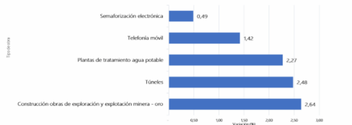
Gráfica 5. ICOCIV. Menores variaciones del año corrido, según tipología de obra Total nacional Marzo 2024
