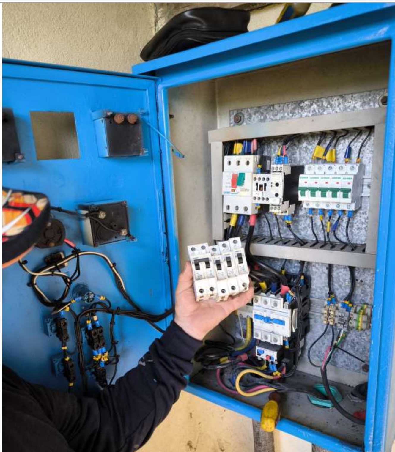
Fotografía Cambio de accesorio tablero de control pozo profundo Dragoncitos
