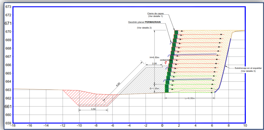
Imagen N° 2. Detalles constructivos muro en tierra armada
