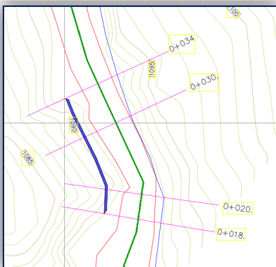
Imagen N° 3. Detalle de la implantación del muro de contención en concreto reforzado sector Las Cruces
