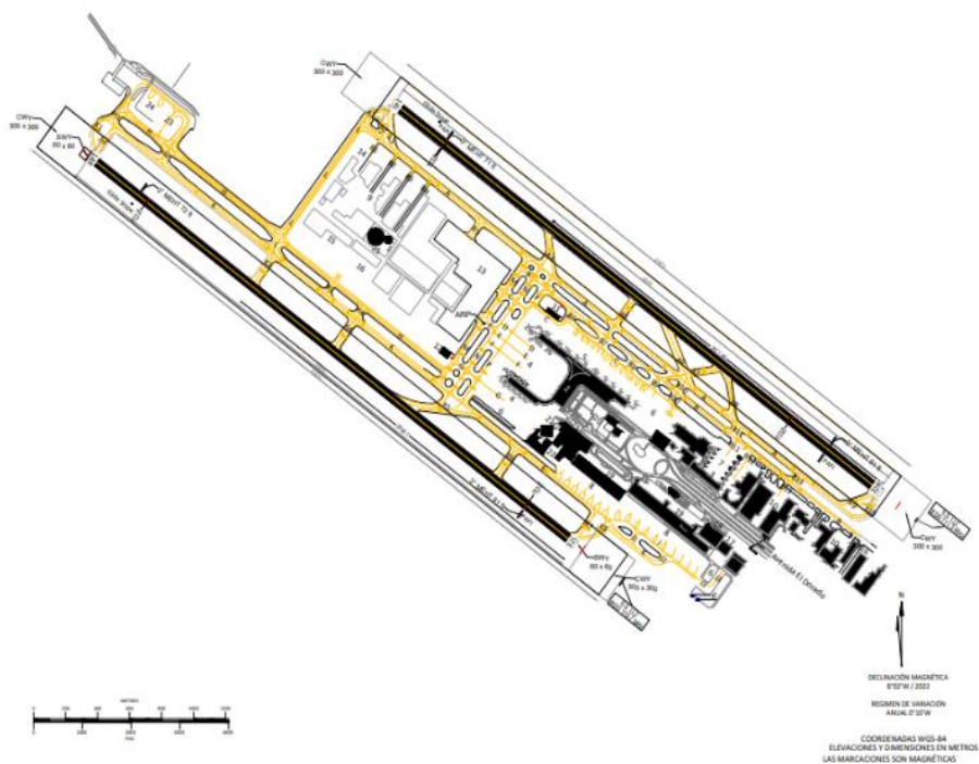
Figura 2. Plano Aeródromo Aeropuerto El Dorado publicado AIP Fuente: AEROCIVIL.
