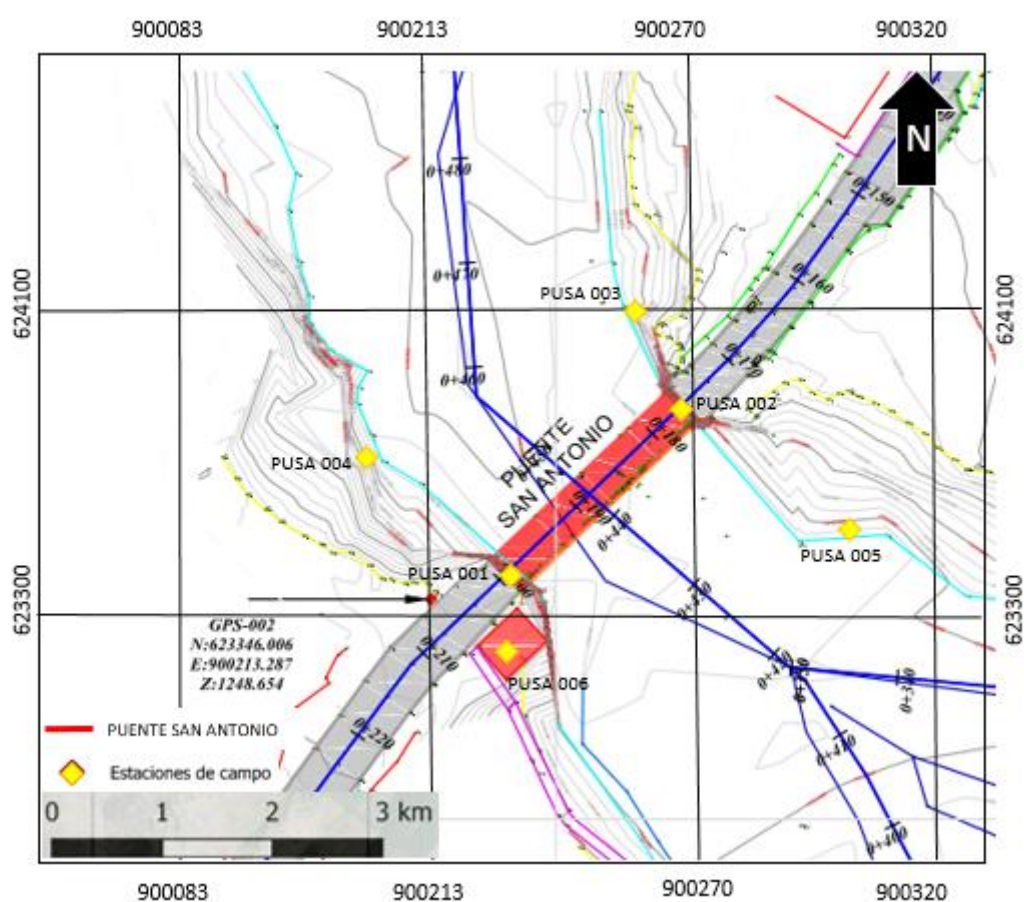
Figura 9 Localización de Puntos de Control en Campo
