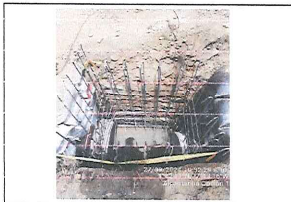
Foto1: armado acero de refuerzo encofe alcantarilla
