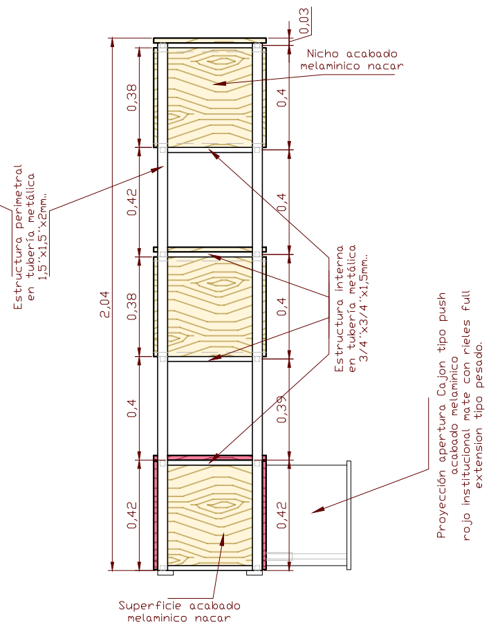
ALZADO LATERAL DERECHO
