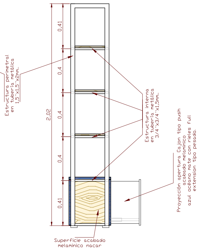
ALZADO LATERAL DERECHO
