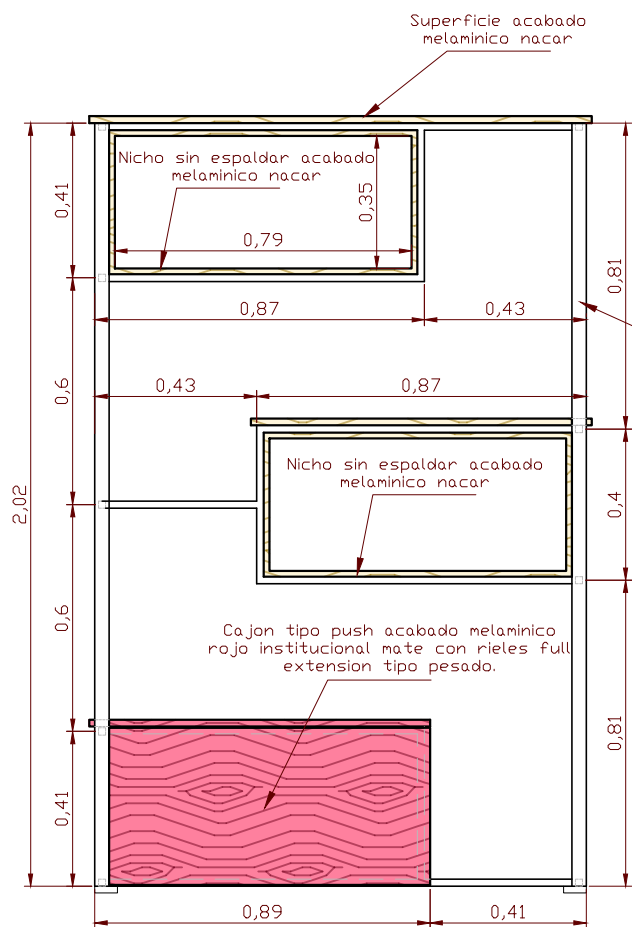
ALZADO FRONTAL
