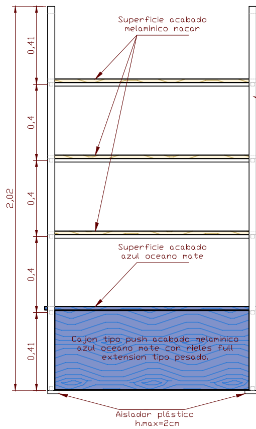
ALZADO FRONTAL
