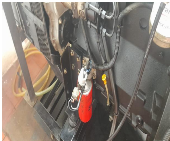
Foto 3. Suministro y cambio de filtro de aceite
