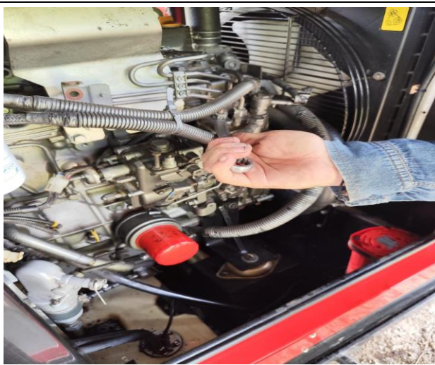
Foto 2. Limpieza de inyectores.
