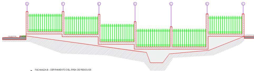
FACAHADA B - CERRAMIENTO DEL ÁREA DE RESIDUOS SENA SECC. 10 Escala Gráfica (m)
