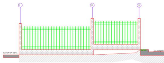
FACAHADA C - CERRAMIENTO DEL ÁREA DE RESIDUOS SENA SECC. 10 Escala Gráfica (m)
