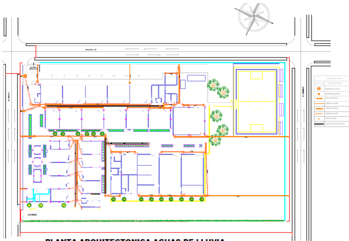
PLANTA ARQUITECTONICA AGUAS DE LLUVIA
