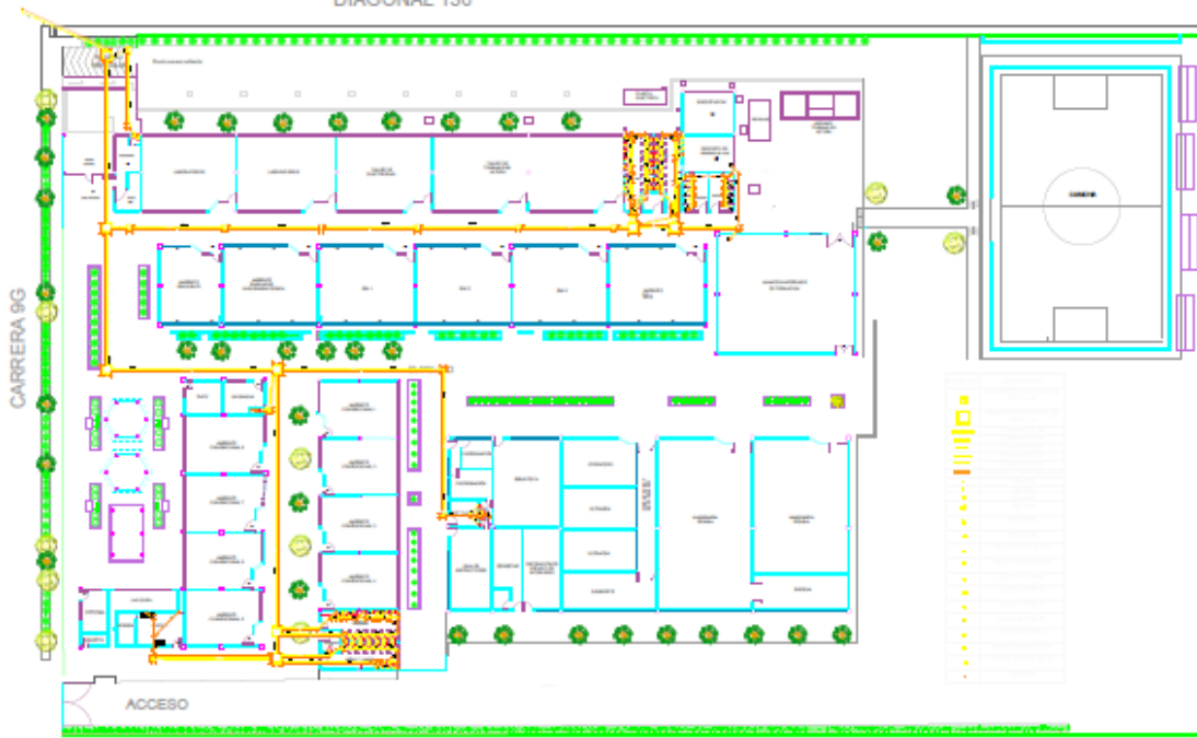
PLANTA DE INSTALACION SANITARIA
