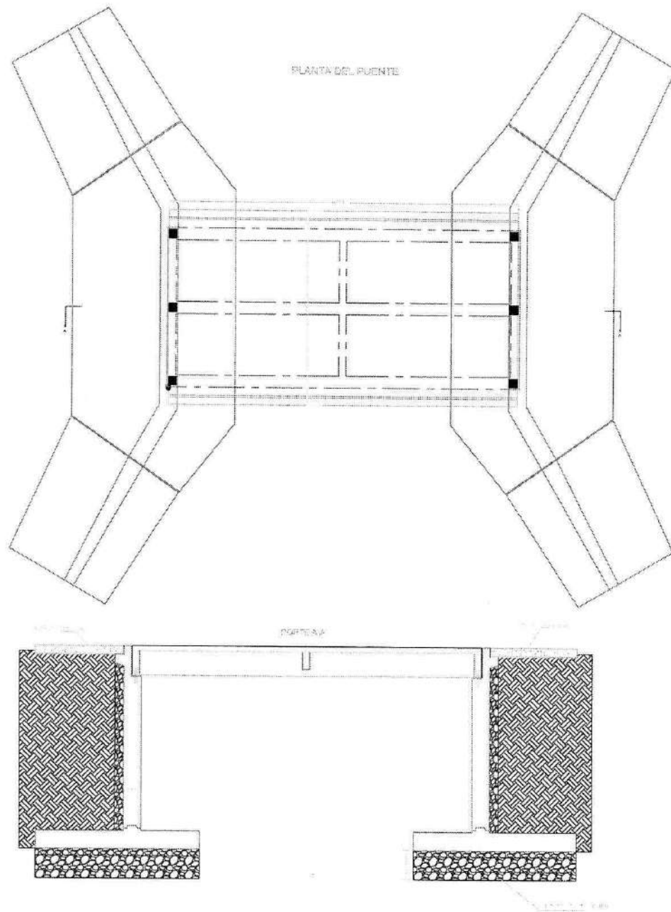
Figura 1. Planta y Sección Transversal del Puente
