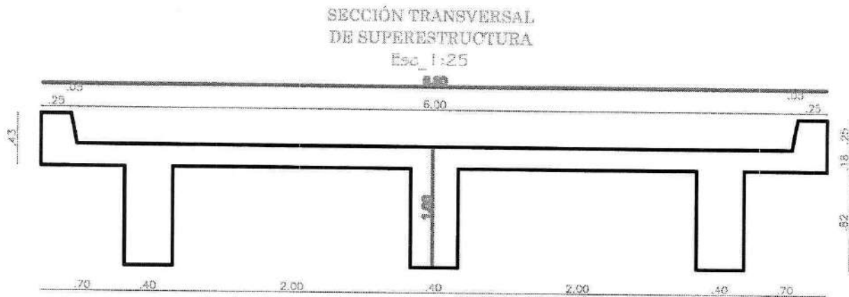
Figura 2. Sección Transversal de la Superestructura
