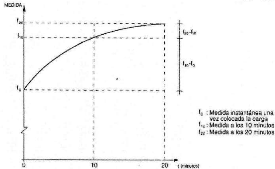
Figura 6. Proceso de carga. Obtenido de Recomendaciones para la realización de pruebas de carga de recepción en puente de carretera, España.
