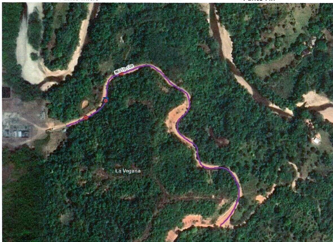
ILUSTRACIÓN 22 UBICACIÓN DEL EJE DE LA VÍA 85010-109 SOBRE IMAGEN SATELITAL DE LA PLATAFORMA ARCGIS
