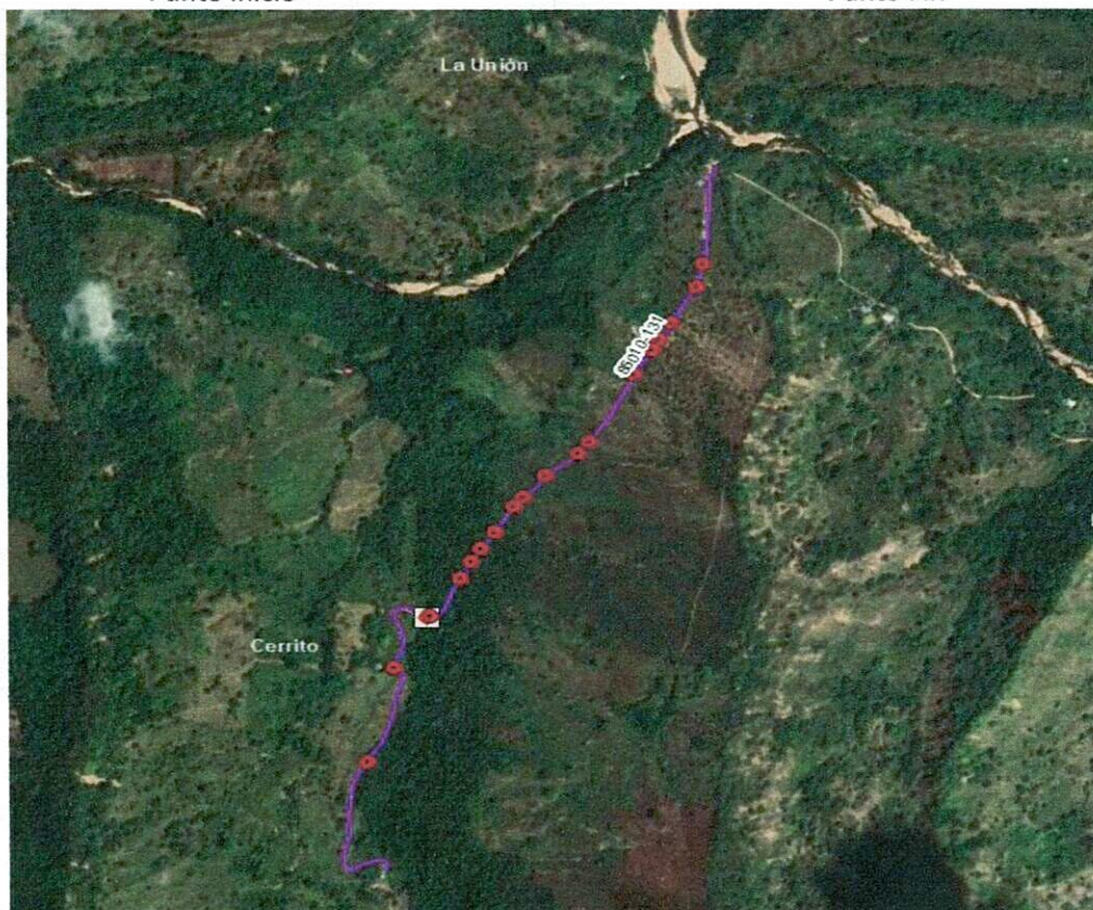
ILUSTRACIÓN 38 UBICACIÓN DEL EJE DE LA VÍA 85010-131 SOBRE IMAGEN SATELITAL DE LA PLATAFORMA ARCGIS
