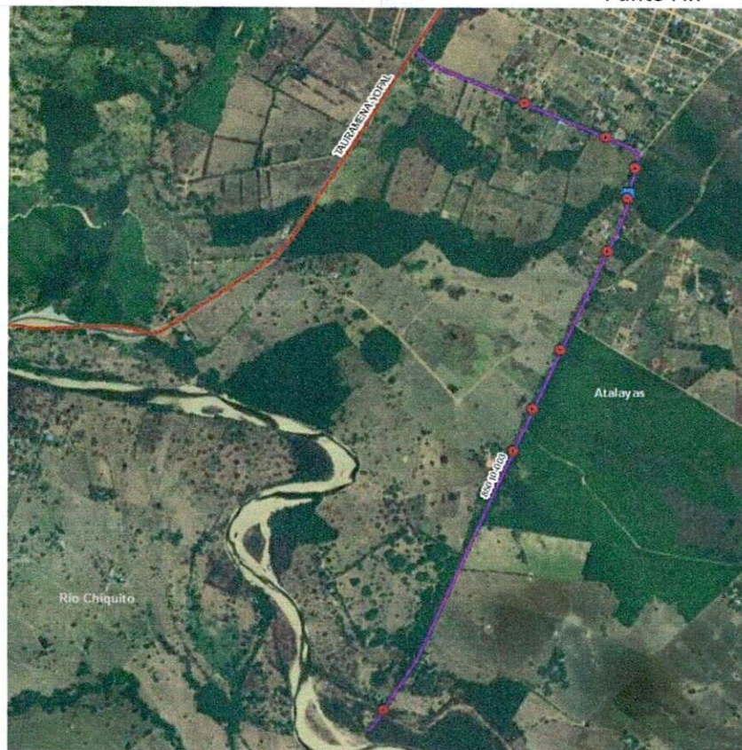
ILUSTRACIÓN 4 UBICACIÓN DEL EJE DE LA VÍA 85010-003 SOBRE IMAGEN SATELITAL DE LA PLATAFORMA ARCGIS
