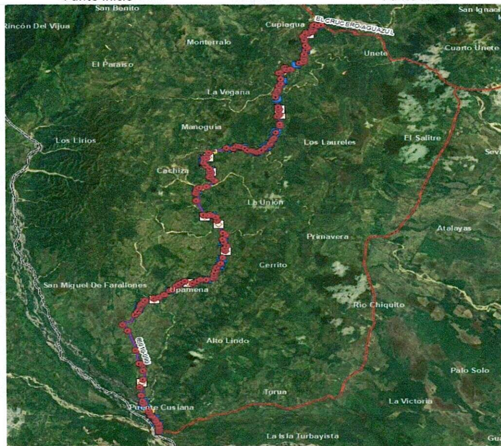
ILUSTRACIÓN 15 UBICACIÓN DEL EJE DE LA VÍA 85010-090 SOBRE IMAGEN SATELITAL DE LA PLATAFORMA ARCGIS
