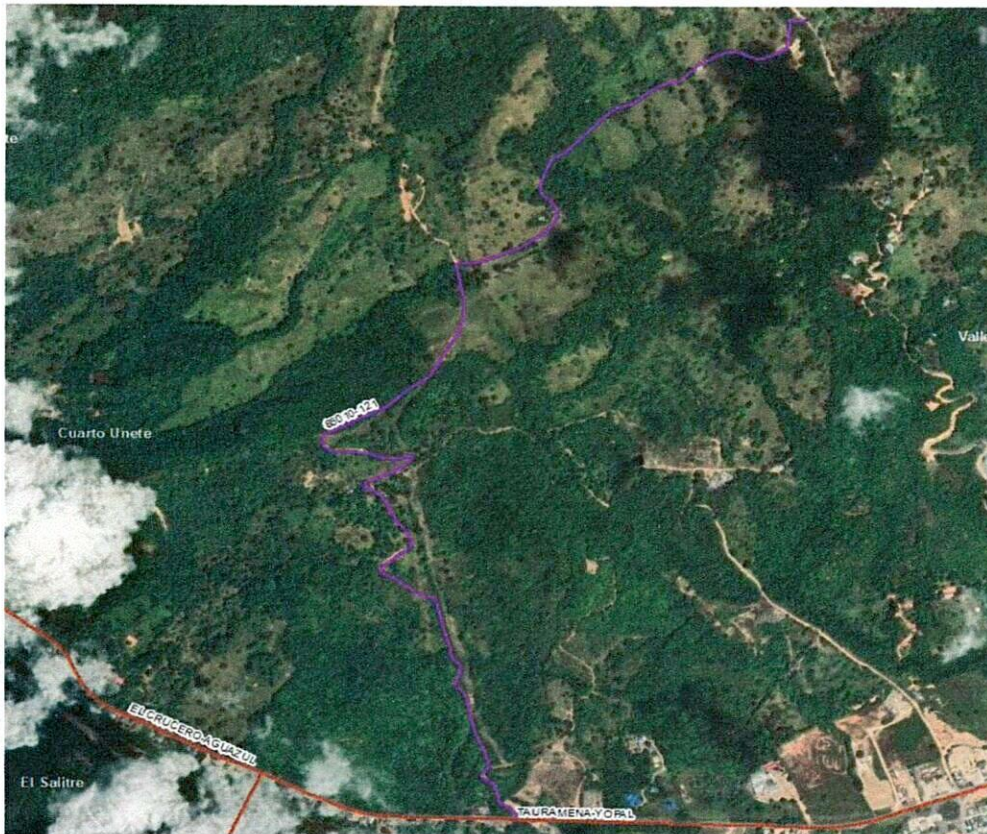
ILUSTRACIÓN 30 UBICACIÓN DEL EJE DE LA VÍA 85010-121 SOBRE IMAGEN SATELITAL DE LA PLATAFORMA ARCGIS
