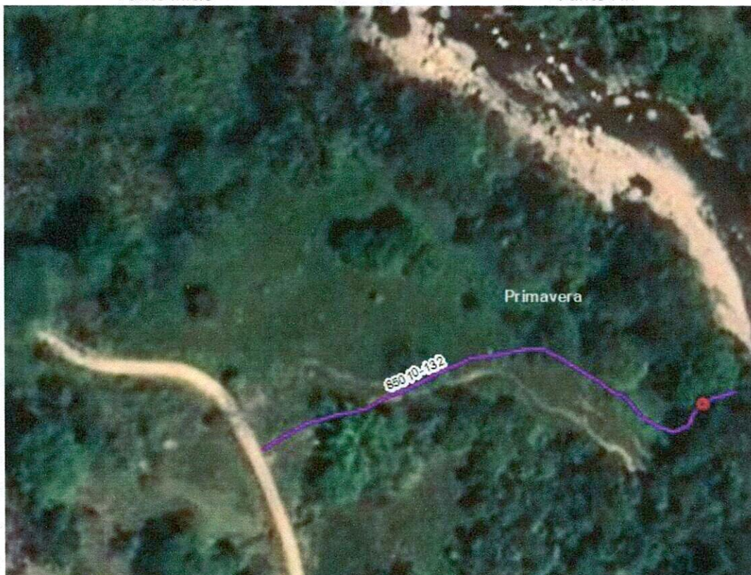
ILUSTRACIÓN 39 UBICACIÓN DEL EJE DE LA VÍA 85010-132 SOBRE IMAGEN SATELITAL DE LA PLATAFORMA ARCGIS
