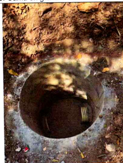
Ilustración 10. construcción de pozo de inspección
