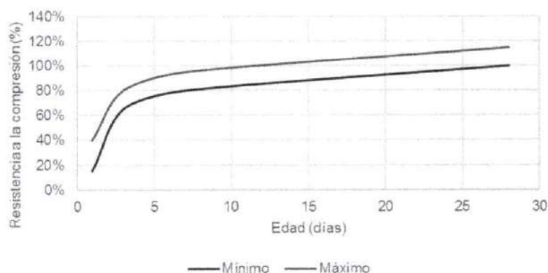
Desarrollo de resistencia en planta Descarga Directa
