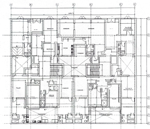
PRIMER NIVEL
