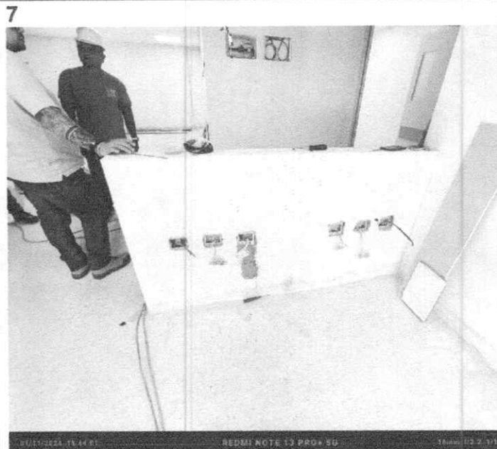
FOTO 4: INSTALACION DE CABLE PARA RED ELECTRICA
