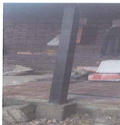
BASES EN CONCRETOCOLUMNAS METALICAS (,25*,25)
