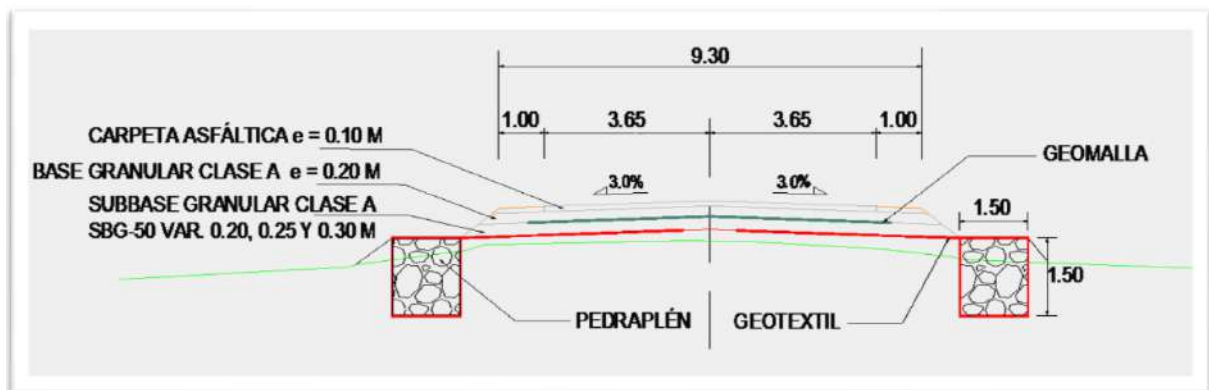
Ilustración 2 Diseño de pavimento flexible
