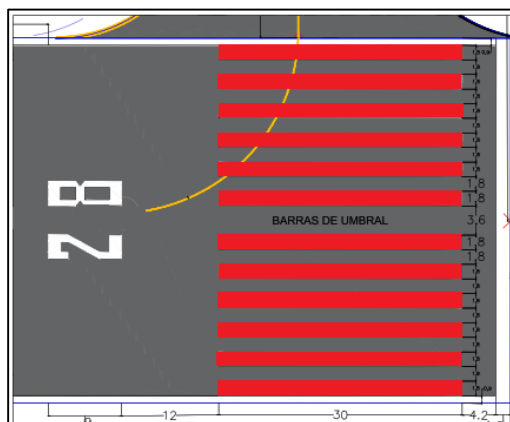
Ilustración 6. Barras de umbral
