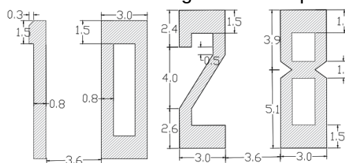
Ilustración 7. Designadores de pista
