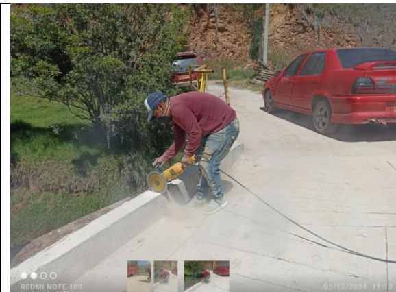
Imagen 7: Corte de dilatación de bordillo k0+010.
