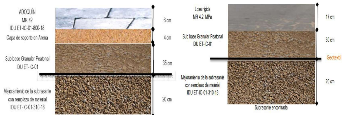
Estructuras de diseños según CBR para andén y calzada.
