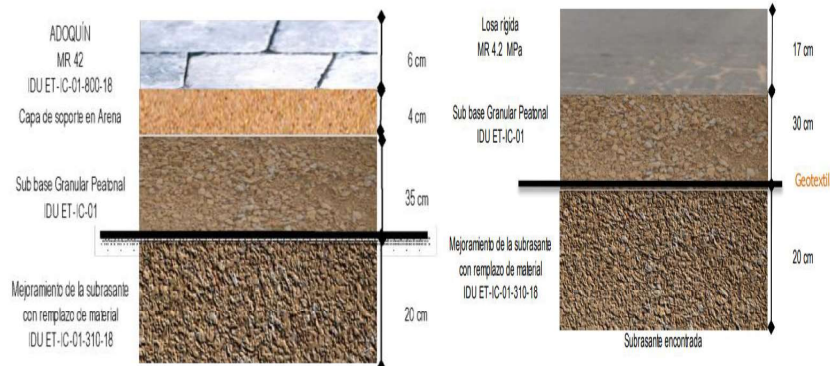
Estructuras de diseños según CBR para andén y calzada.
