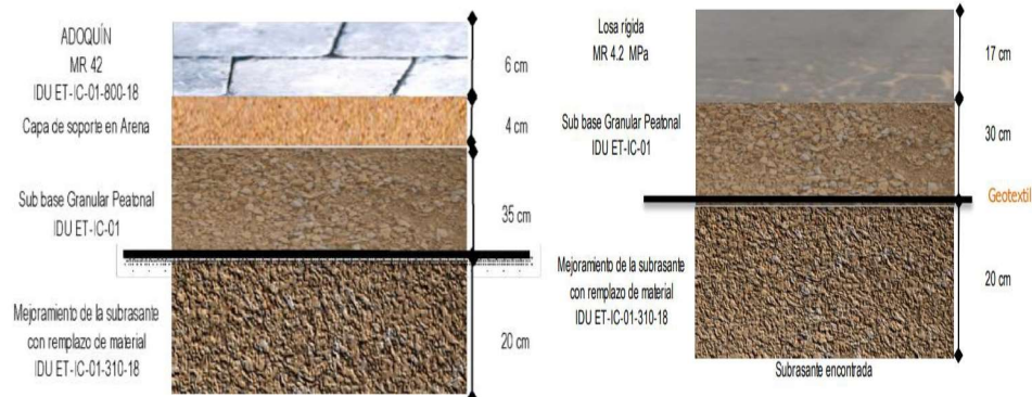
Estructuras de diseños según CBR para andén y calzada
