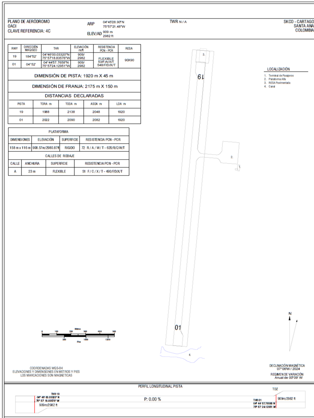
Ilustración 3. Plano de Aeródromo tomado del formato AIP del Aeropuerto Santa Ana de Cartago
